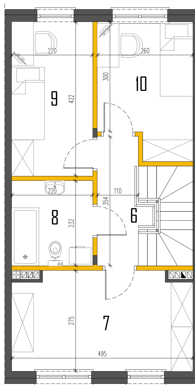
RZUT PIĘTRA
