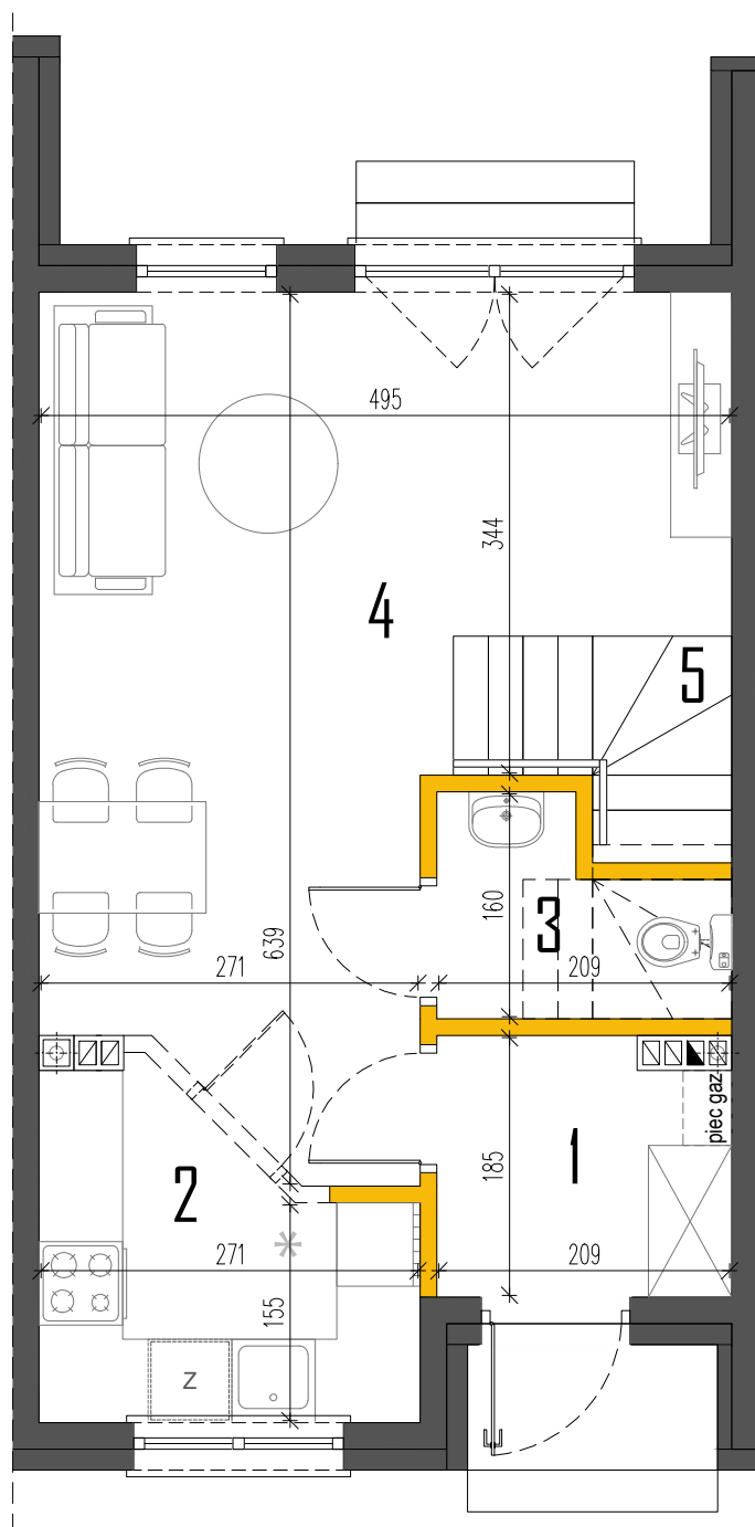
RZUT PARTERU
